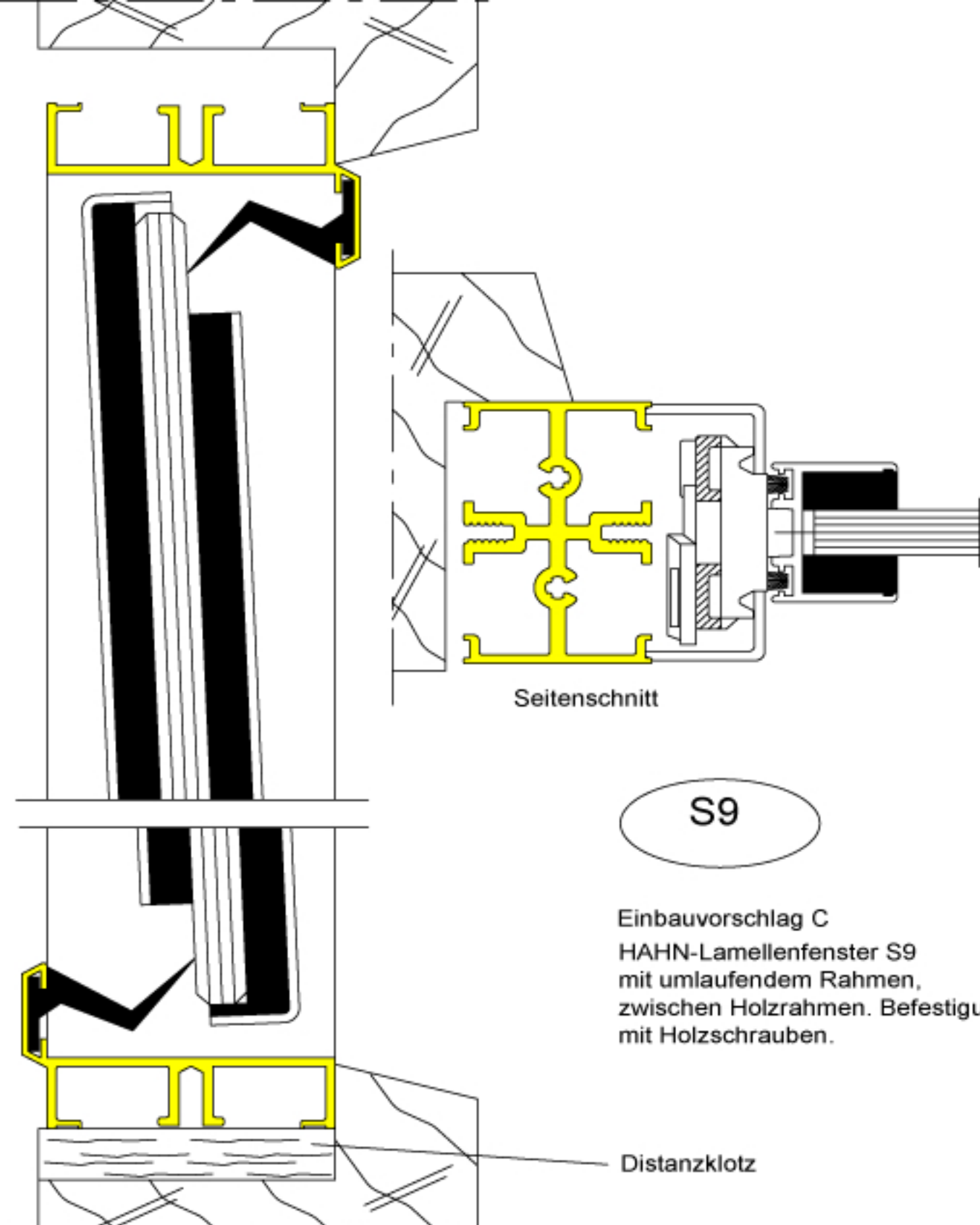
Höhenschnitt M 1:1
